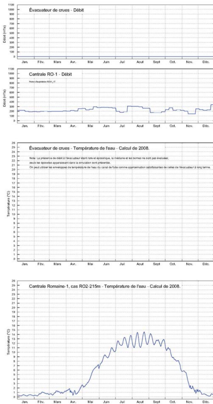
Planche 18. Réservoir Romaine-1. Température de l'eau et débit aux exutoires. Extrait 3 de 21 - Année 1985.
