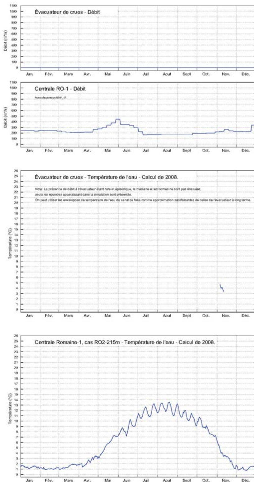
Planche 18. Réservoir Romaine-1. Température de l'eau et débit aux exutoires. Extrait 13 de 21 - Année 1995.
