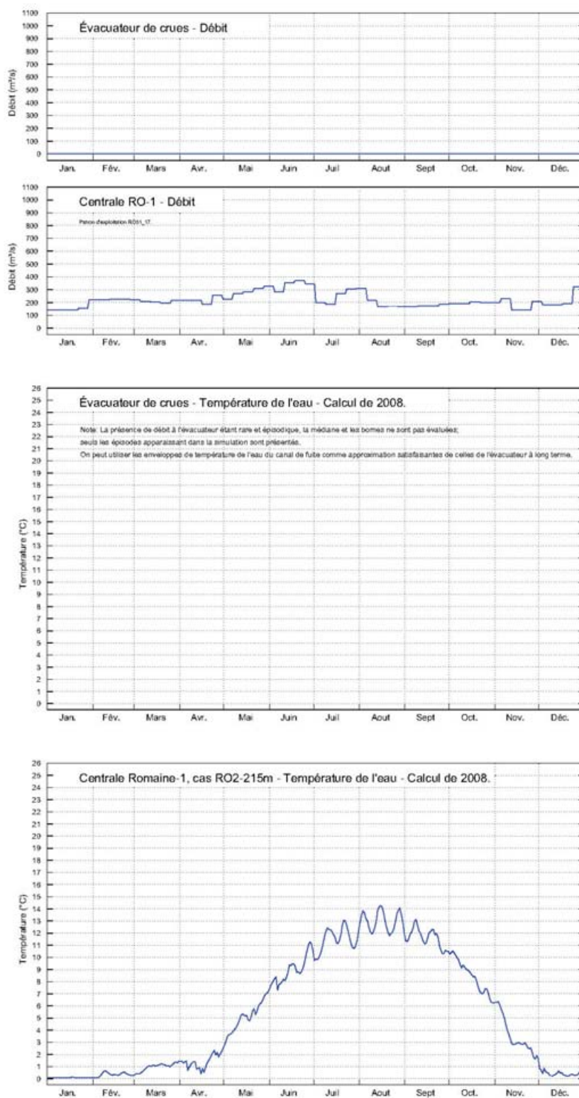
Planche 18. Réservoir Romaine-1. Température de l'eau et débit aux exutoires. Extrait 9 de 21 - Année 1991.
