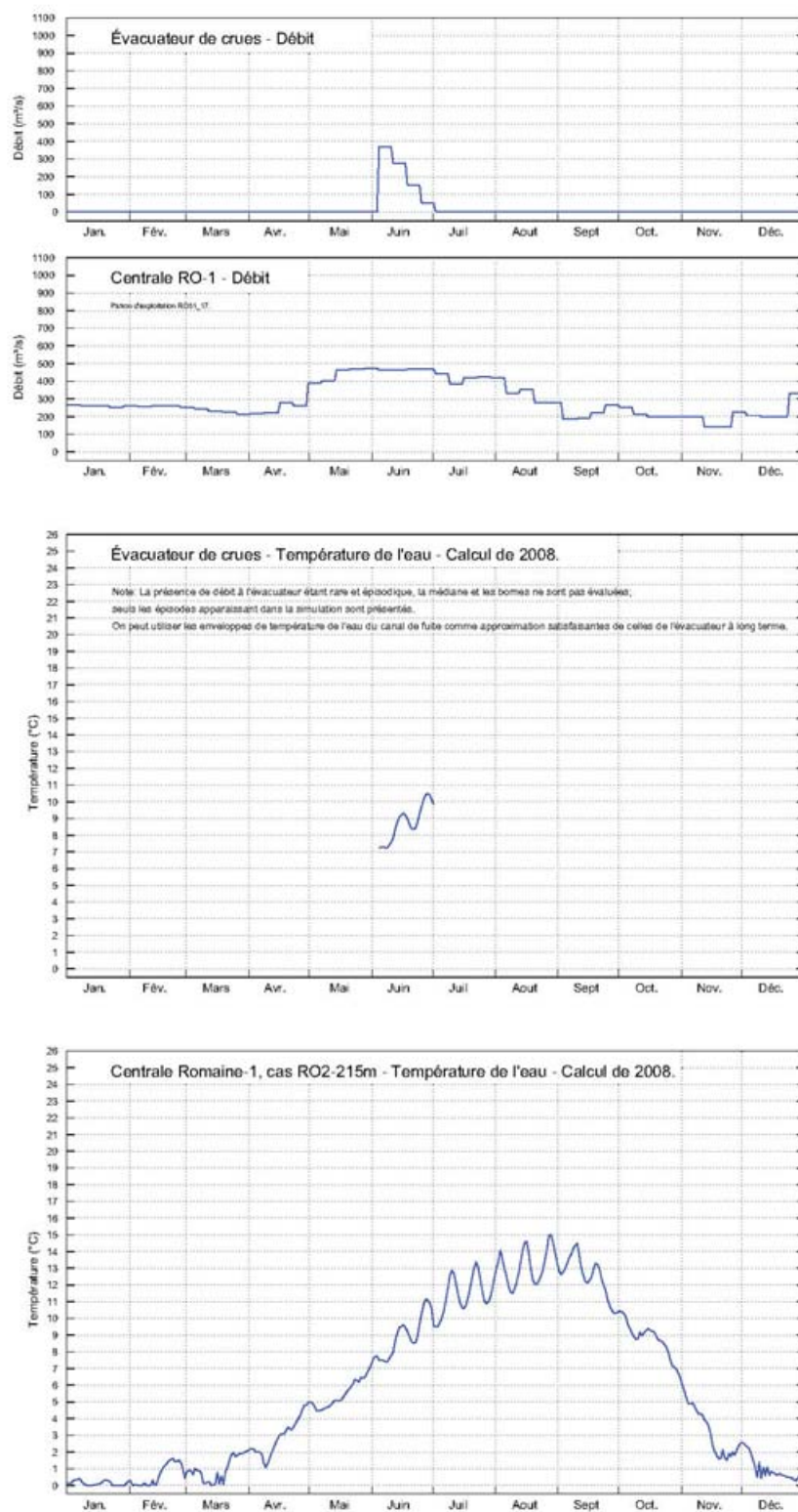
Planche 18. Réservoir Romaine-1. Température de l'eau et débit aux exutoires. Extrait 2 de 21 - Année 1984.
