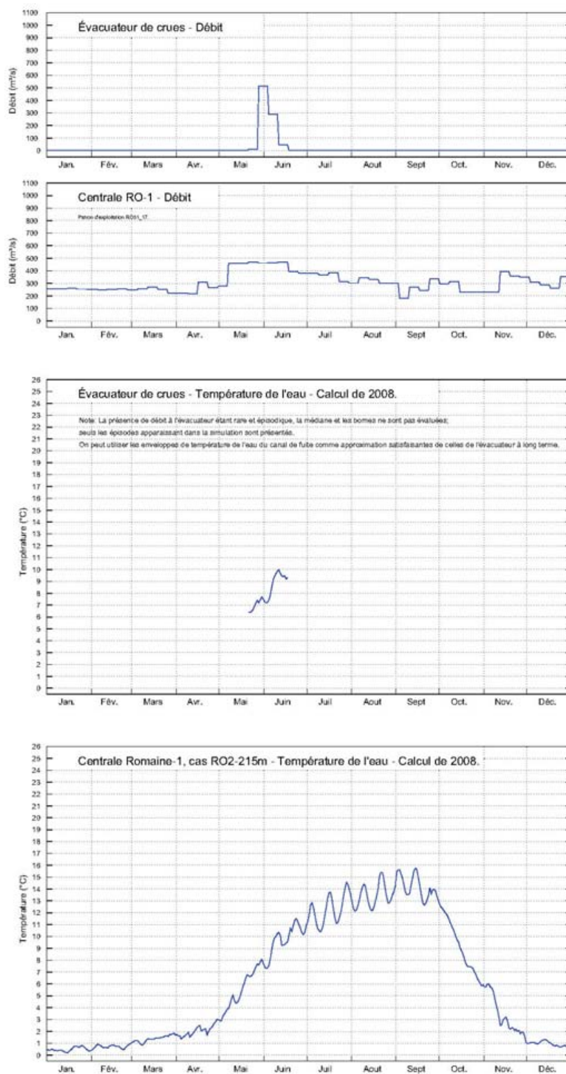
Planche 18. Réservoir Romaine-1. Température de l'eau et débit aux exutoires. Extrait 17 de 21 - Année 1999.
