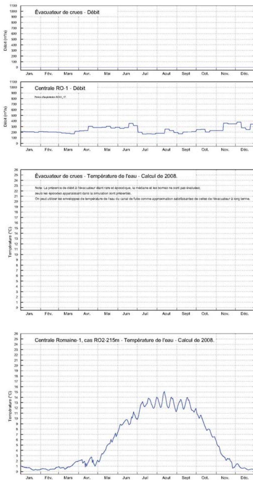
Planche 18. Réservoir Romaine-1. Température de l'eau et débit aux exutoires. Extrait 5 de 21 - Année 1987.
