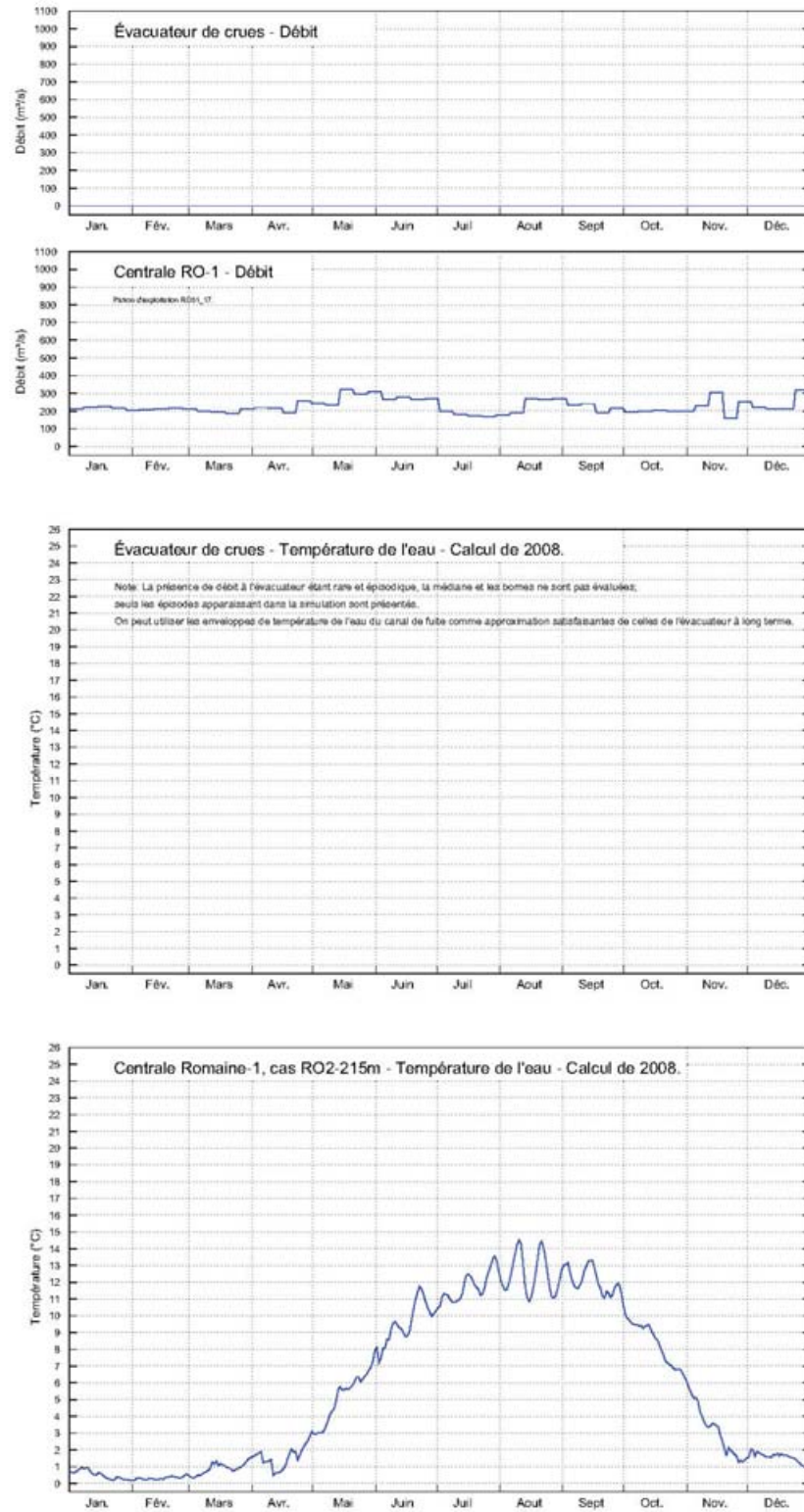
Planche 18. Réservoir Romaine-1. Température de l'eau et débit aux exutoires. Extrait 10 de 21 - Année 1992.
