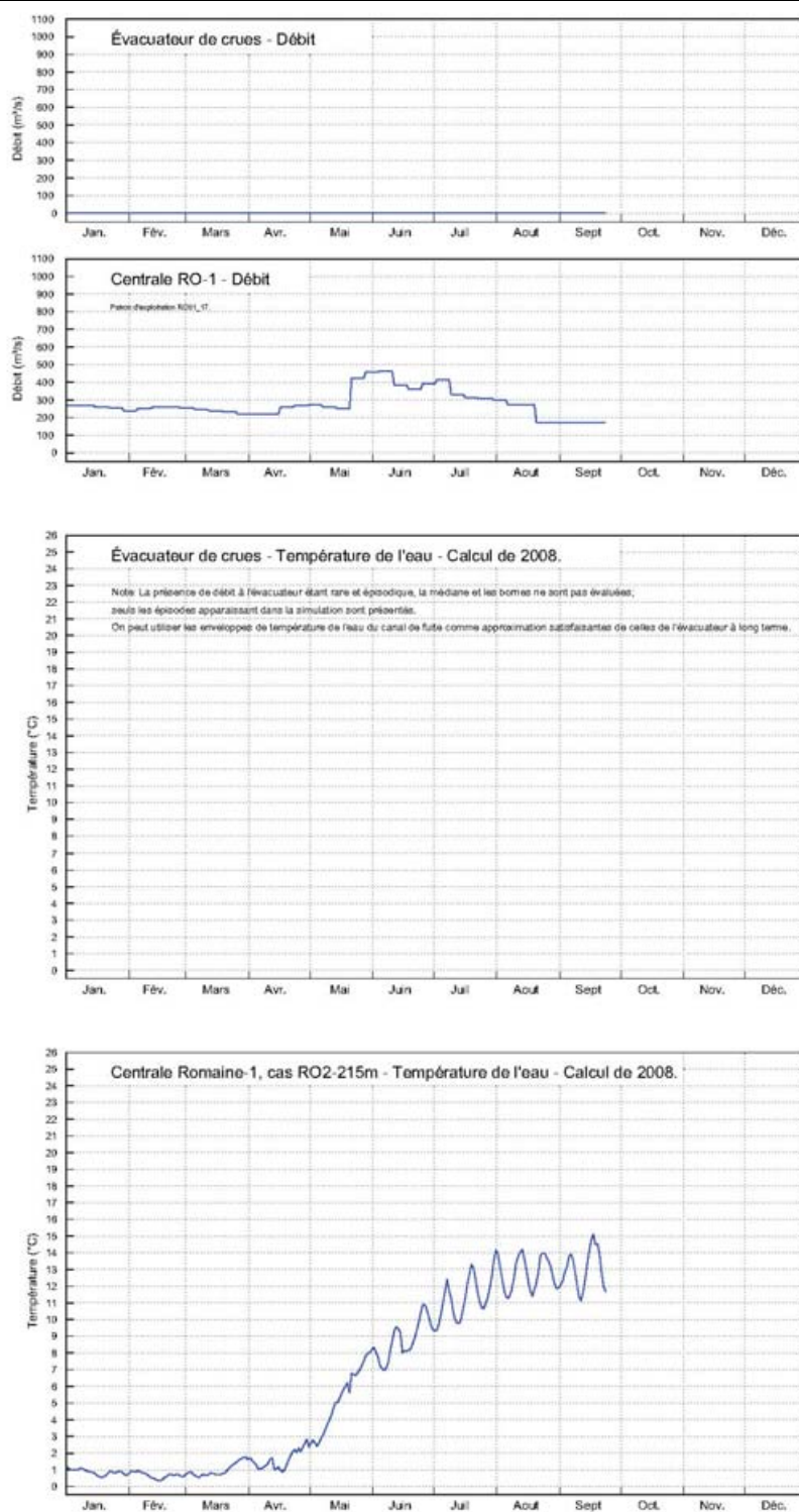
Planche 18. Réservoir Romaine-1. Température de l'eau et débit aux exutoires. Extrait 21 de 21 - Année 2003.
