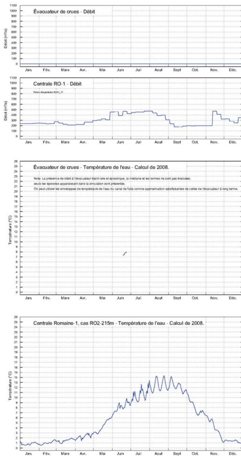
Planche 18. Réservoir Romaine-1. Température de l'eau et débit aux exutoires. Extrait 14 de 21 - Année 1996.
