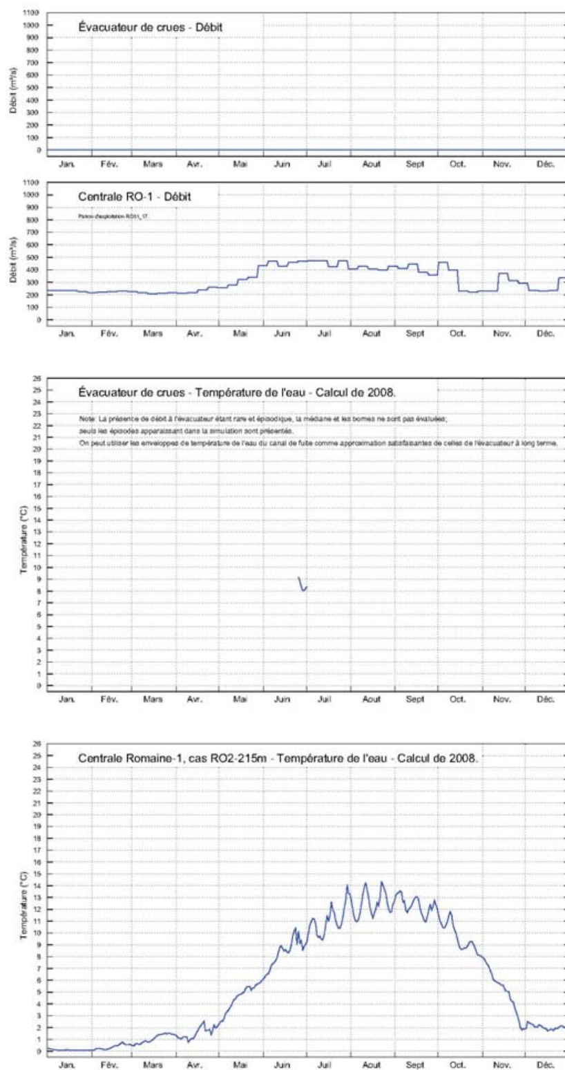
Planche 18. Réservoir Romaine-1. Température de l'eau et débit aux exutoires. Extrait 12 de 21 - Année 1994.
