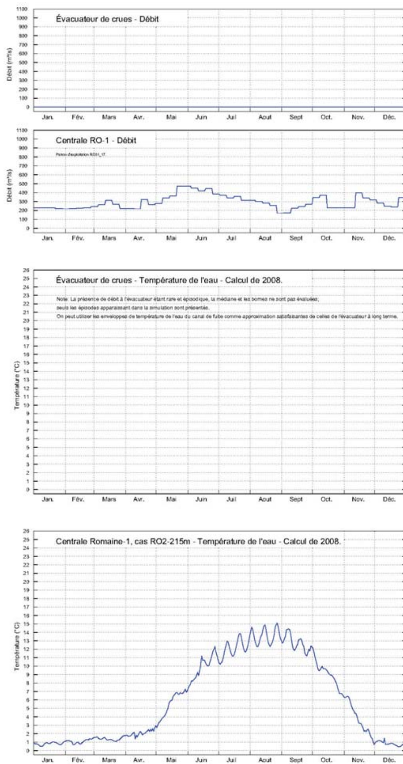
Planche 18. Réservoir Romaine-1. Température de l'eau et débit aux exutoires. Extrait 16 de 21 - Année 1998.
