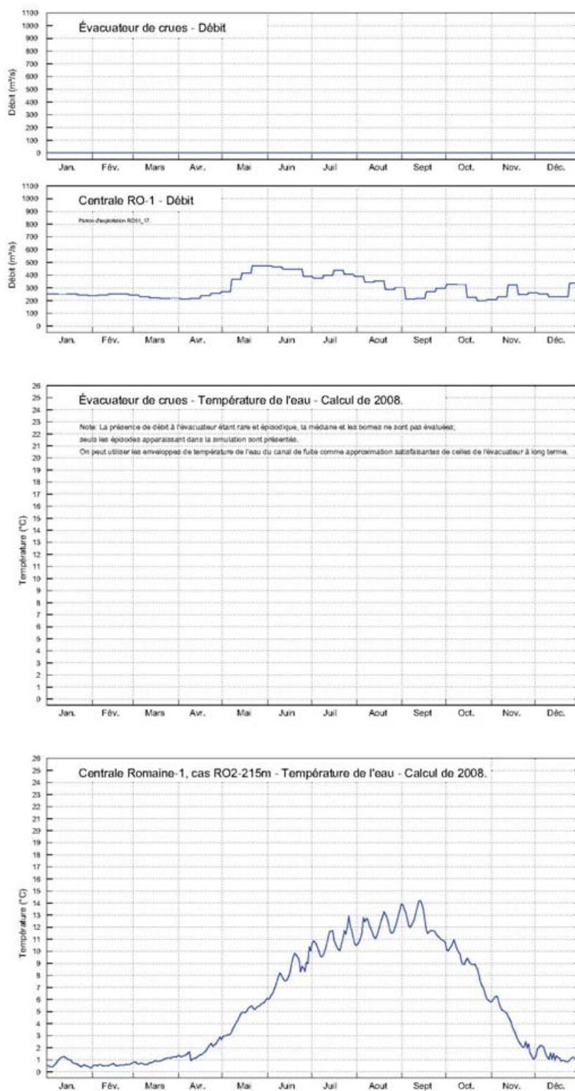
Planche 18. Réservoir Romaine-1. Température de l'eau et débit aux exutoires. Extrait 15 de 21 - Année 1997.
