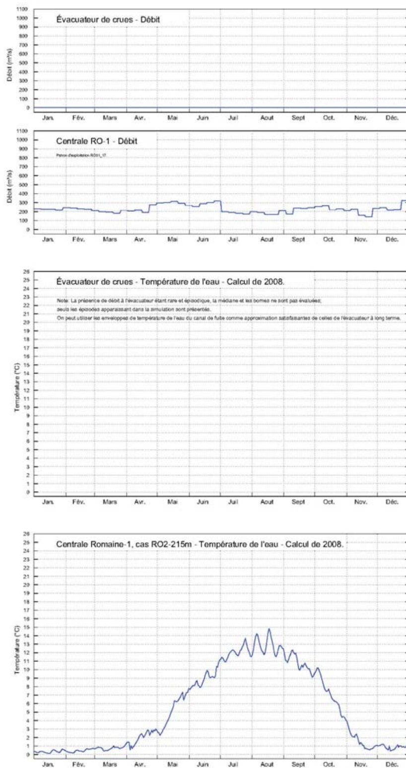
Planche 18. Réservoir Romaine-1. Température de l'eau et débit aux exutoires. Extrait 4 de 21 - Année 1986.
