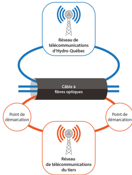
Figure 2 Séparation physique des fibres optiques
