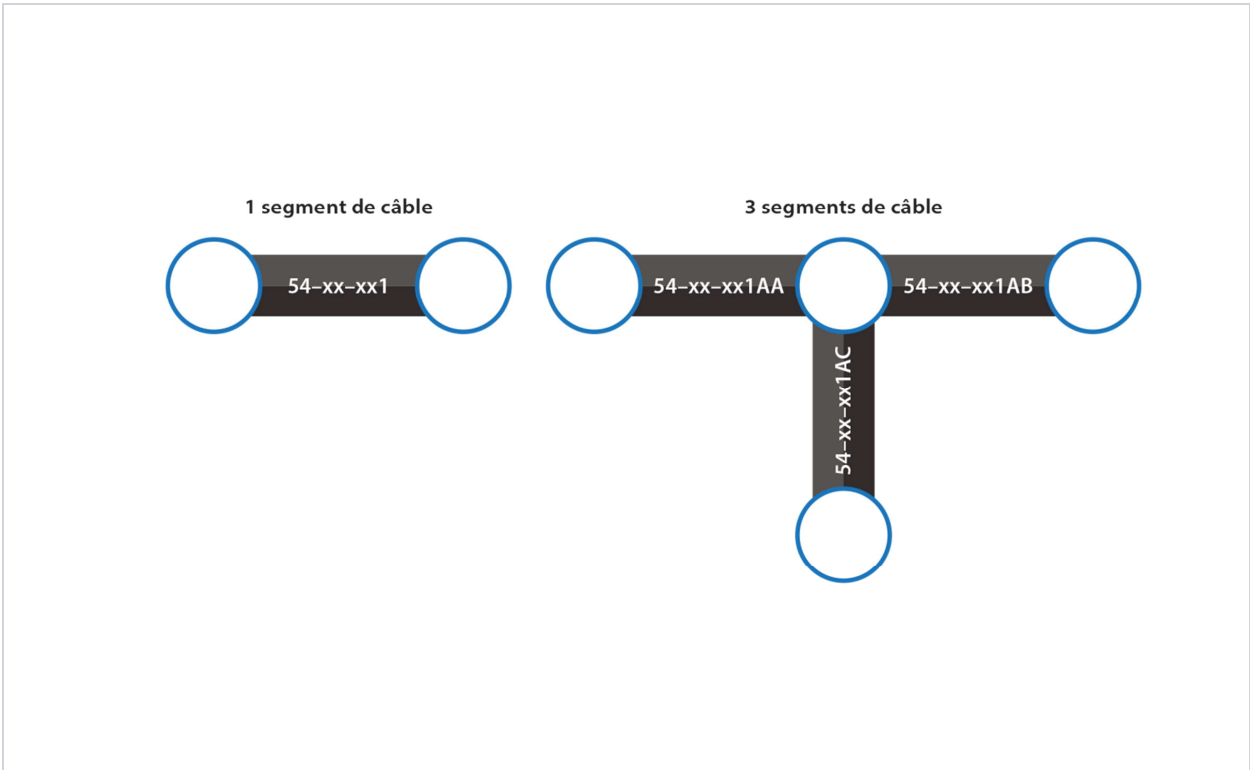
Figure 6 Segmentation d’un câble à fibres optiques
