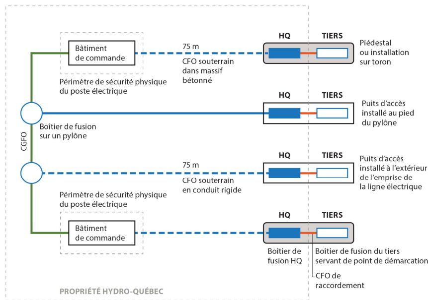
Figure 9 Exemple d'arrangement normalisé pour l'accès à la capacité excédentaire par un tiers
