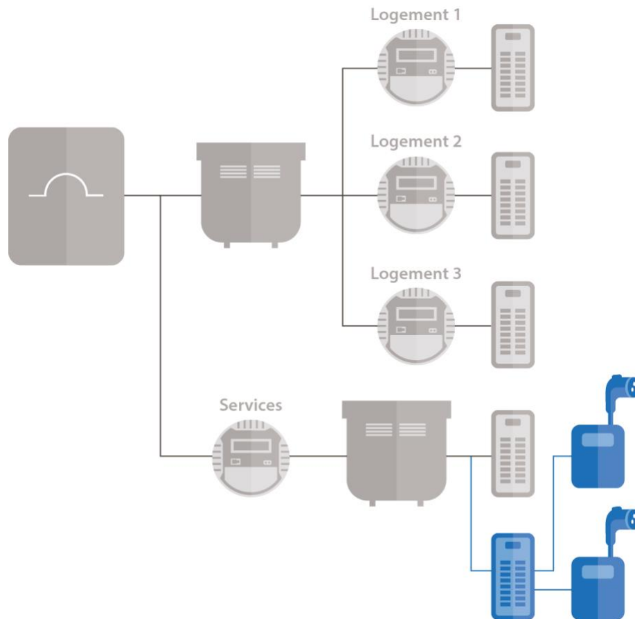
Figure 6 : Nouveau tableau de distribution
