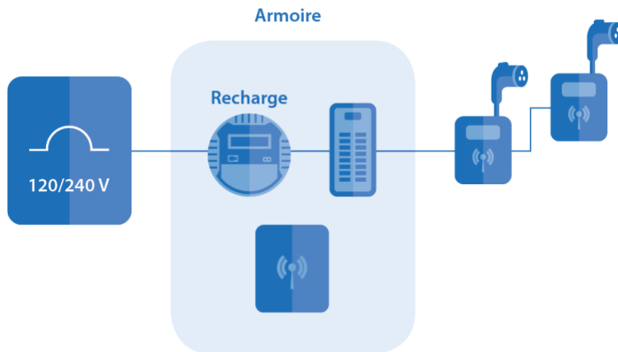
Figure 13 : Raccordement par l'intermédiaire d'une armoire
