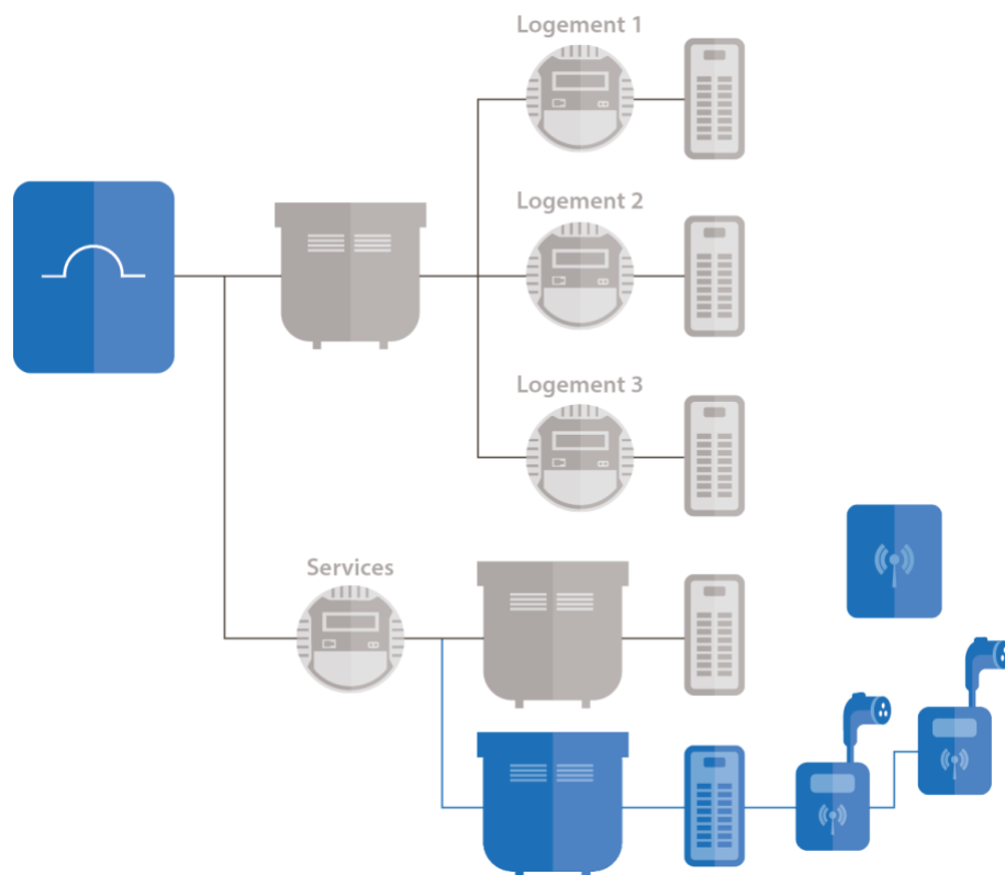
Figure 10 : Raccordement avec gestion de la puissance
