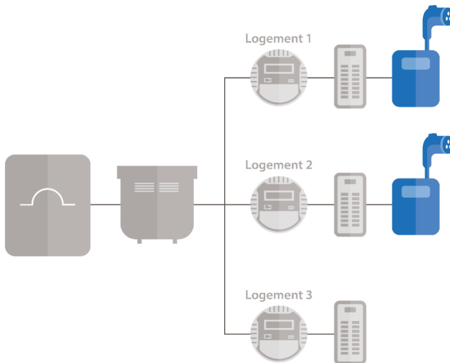
Figure 3 : Raccordement au tableau de distribution électrique
