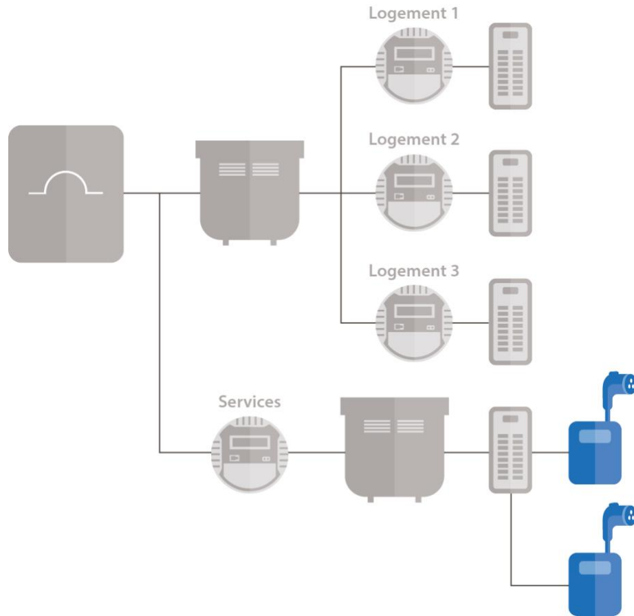
Figure 5 : Raccordement au tableau de distribution des service généraux
