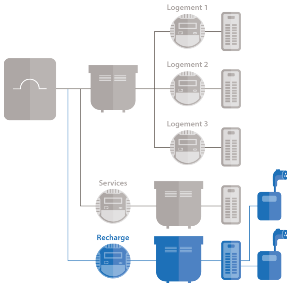
Figure 8 : Compteur réservé à la recharge
