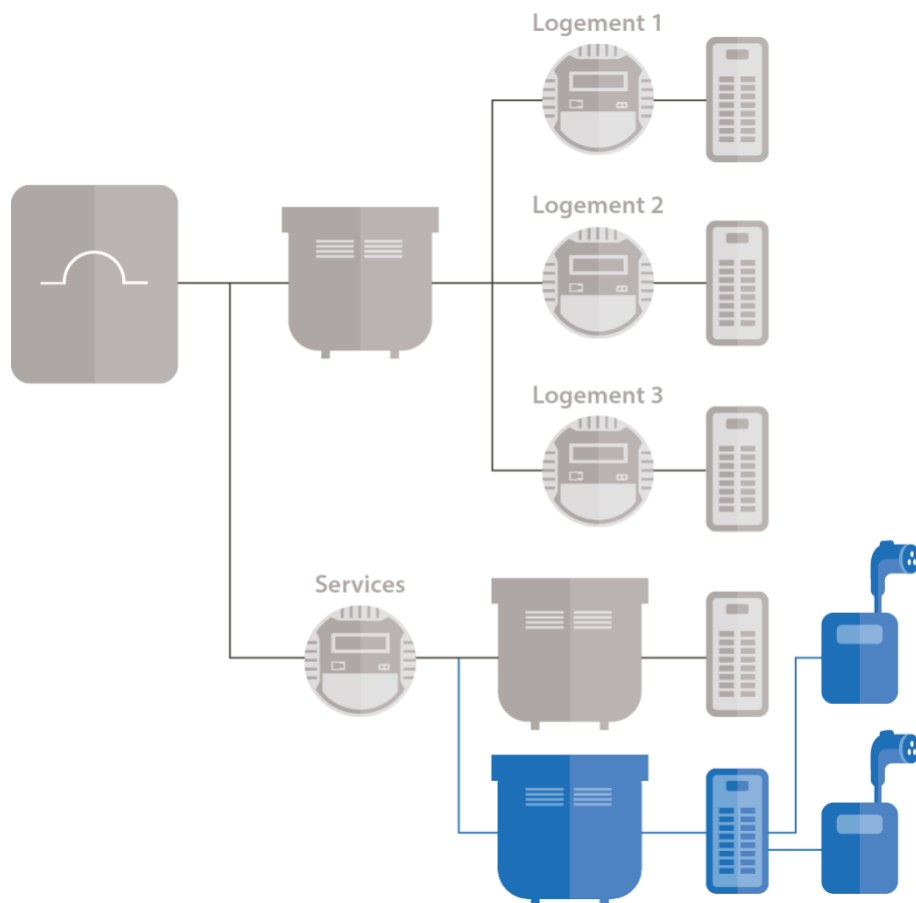
Figure 7 : Nouveau transformateur
