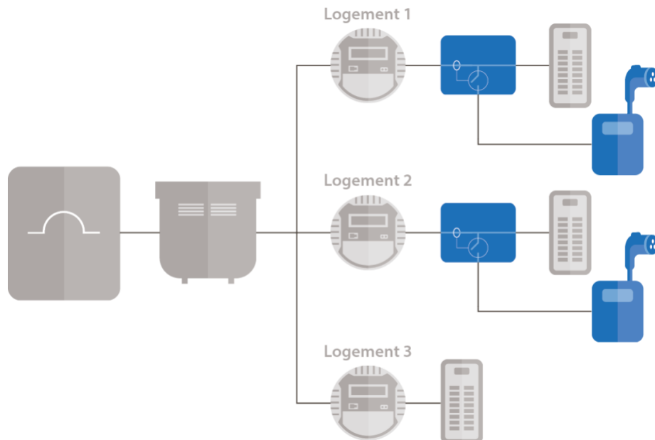
Figure 4 : Raccordement à un contrôleur de charge
