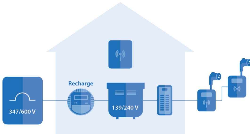
Figure 12 : Raccordement par l'intermédiaire d'un bâtiment de service
