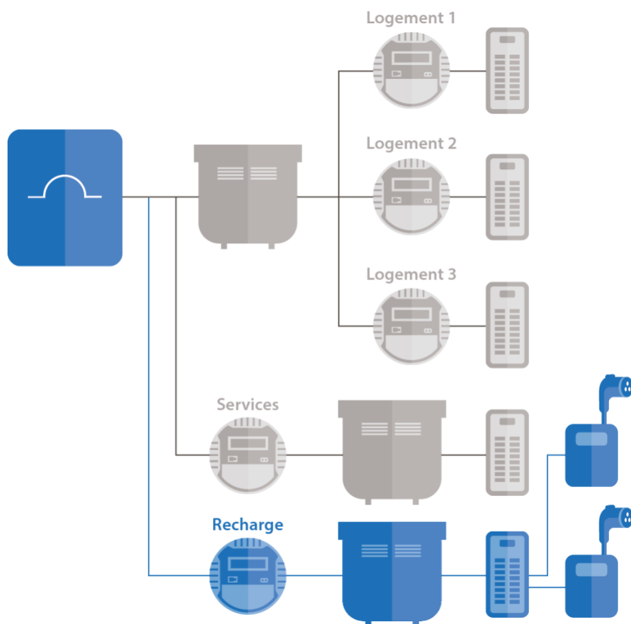
Figure 9 : Nouveau branchement du client
