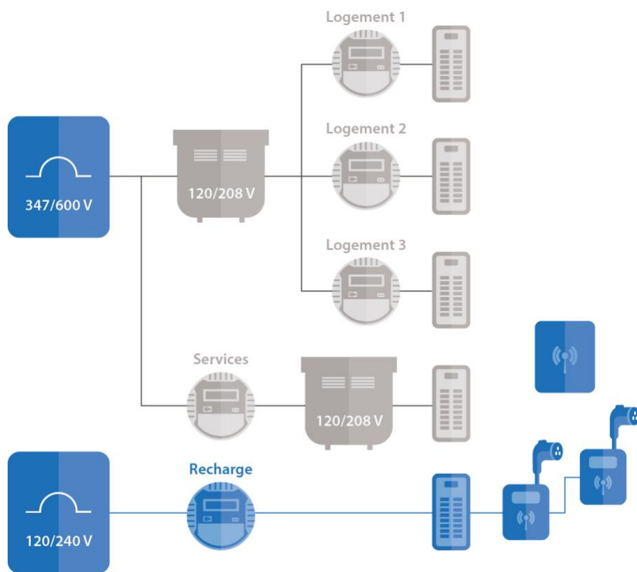
Figure 11 : Raccordement à un branchement à une tension différente
